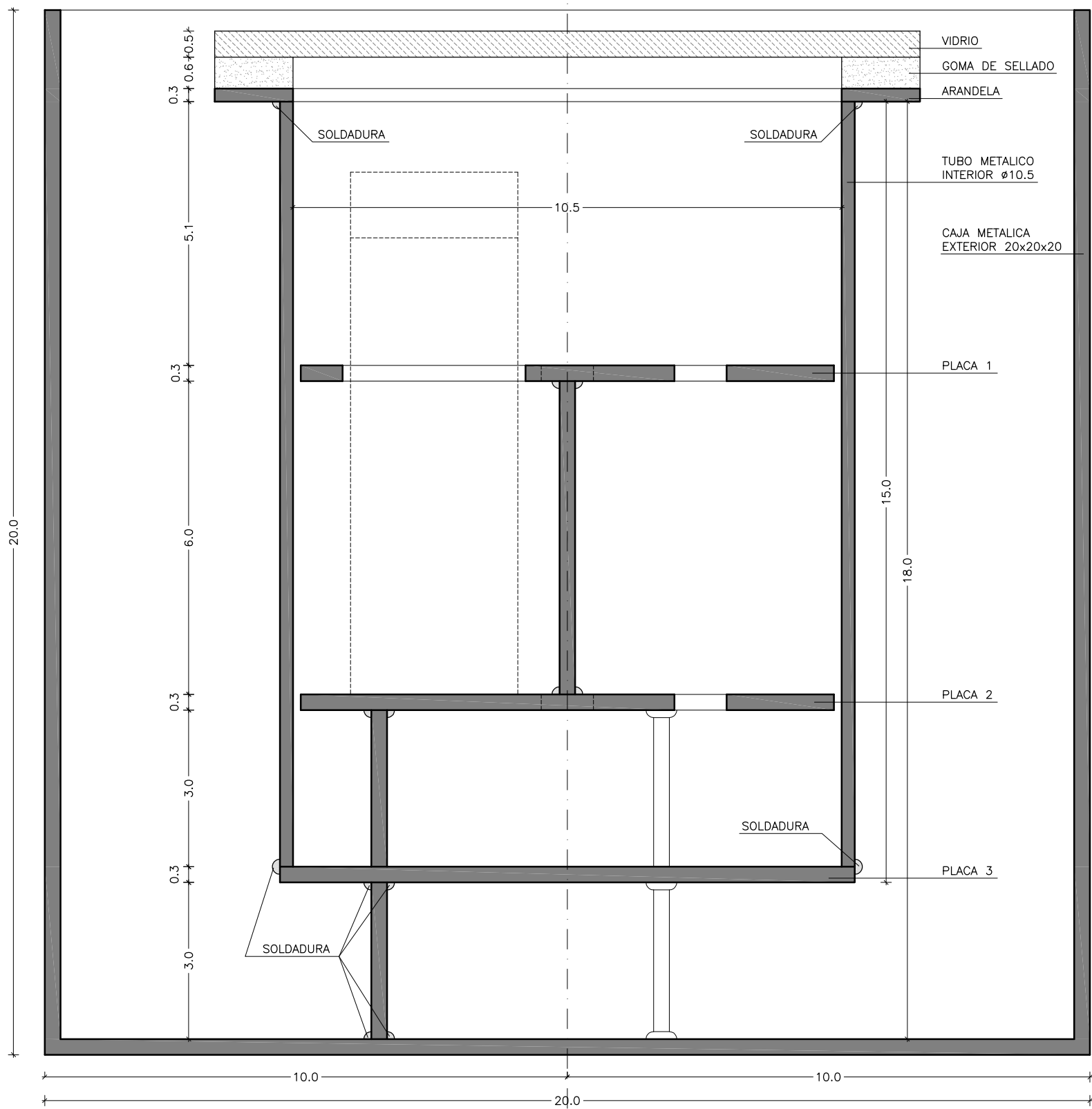
SECCION B-B
